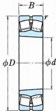
錐形孔
