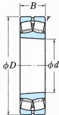
錐形孔
